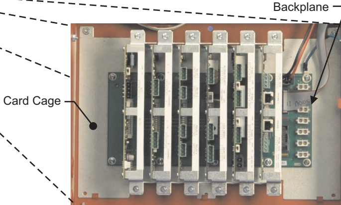
Backplane
